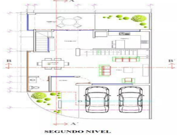
SEGUNDO NIVEL
