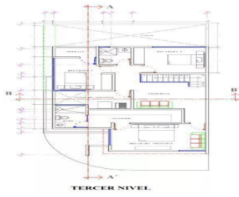
TERCER NIVEL
