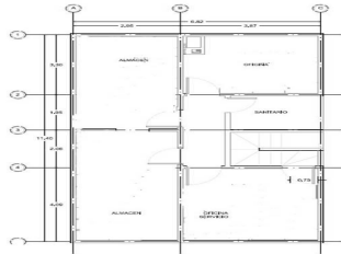
PLANO ARQUITECTONICO 1ER NIVEL esc. 1:50 cot. metros
